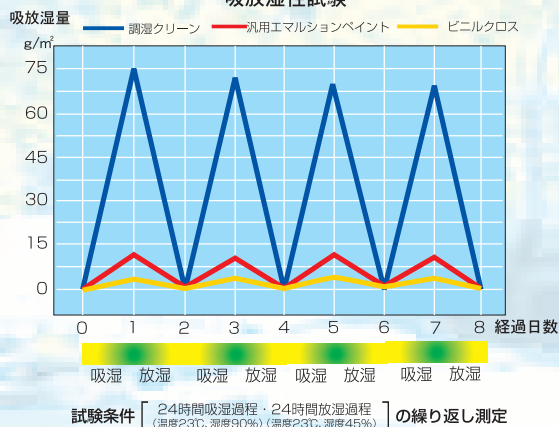
吸放湿性試験
