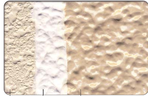
旧塗膜 エスケー弾性プレミアムフィラー エスケープレミアムシリコン等
